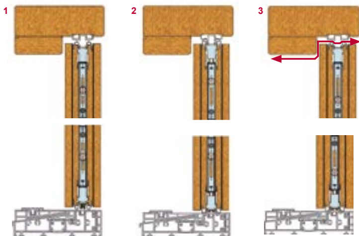
Ilustracja 1 okucie i skrzydło w pozycji jezdnej
